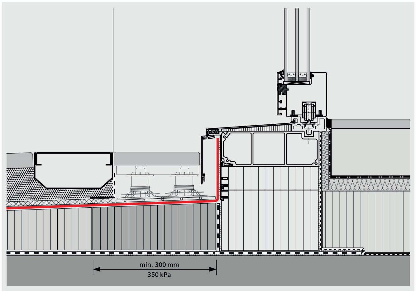
Figure 5.141 : Caniveau sur couche d'usure à joints fermés sur la ligne de fuite de la façade avec zone de couverture à joints ouverts près de la fenêtre.
