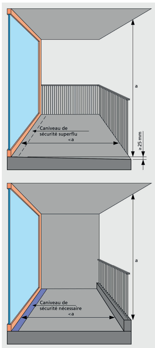
Figure 5.143: Sur les balcons et coursives avec une hauteur de déversement libre sur la longueur et se situant 25 mm sous le raccord au seuil, on peut renoncer à un caniveau de sécurité, mais pas si la hauteur de déversement est rehaussée.
