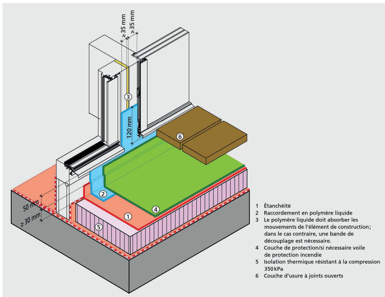
Figure 5.136: Seuils de porte et de fenêtre avec dilatation.
