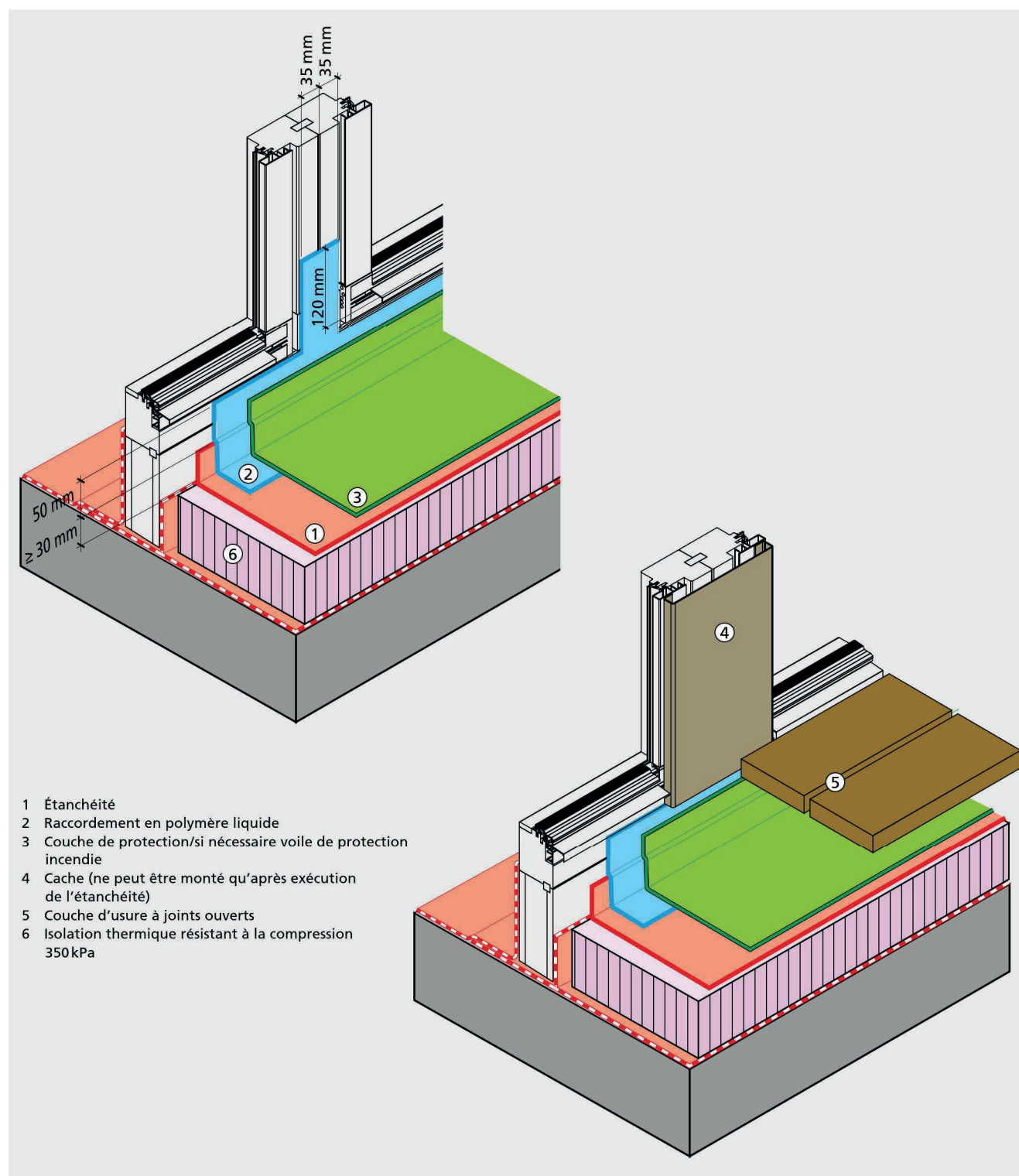
Figure 5.135: Seuils de porte et de fenêtre fixes.
