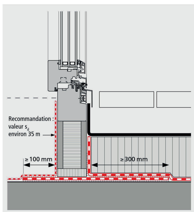
Figure 5.137: Raccordement au pare-vapeur des éléments de porte et de fenêtre.
