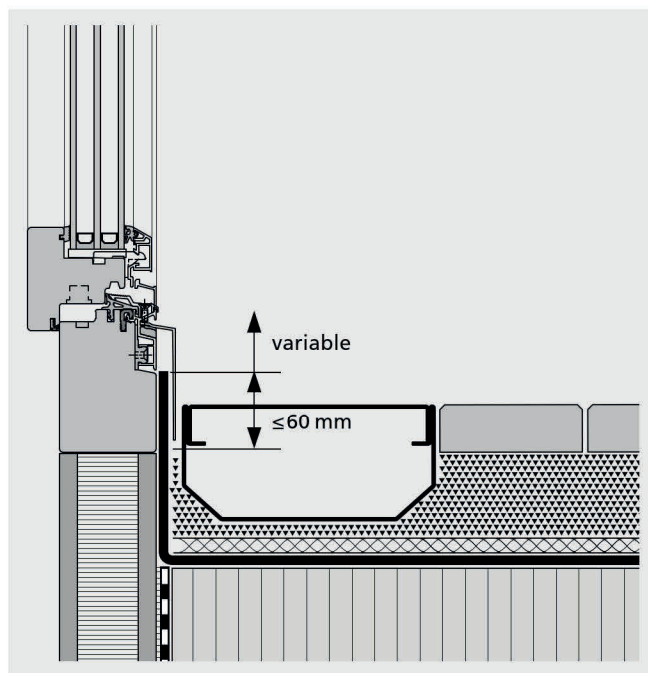
Figure 5.139: Conformément à la norme SIA 271, la largeur des cadres en bois ne doit pas excéder 80 mm, le cadre ne pouvant pas dépasser 60 mm sous le bord supérieur du polymère liquide. Le cadre en bois peut aussi être plus élevé vers le haut.
