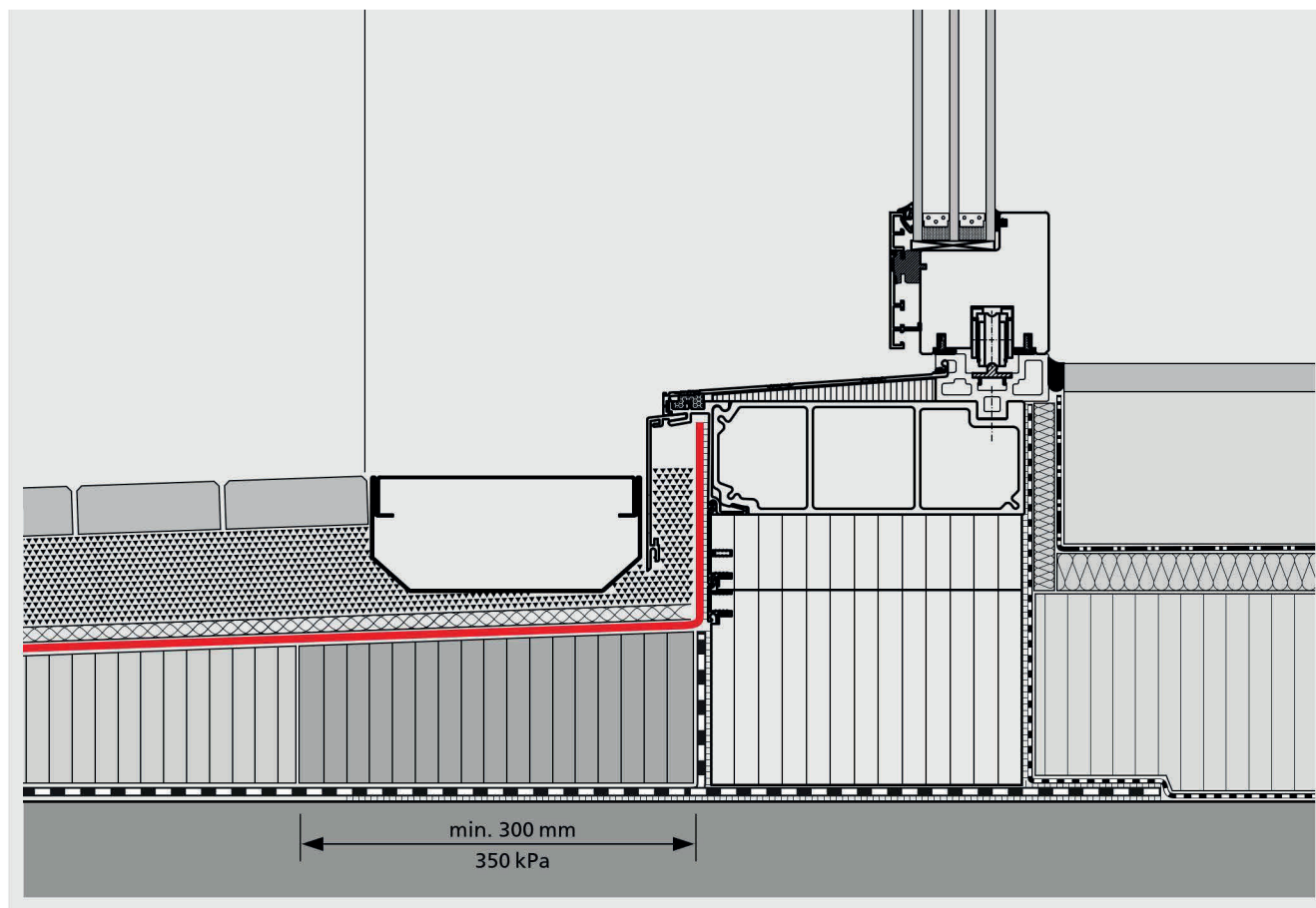
Figure 5.140: Caniveau devant le seuil sur couche d'usure à joints fermés.
