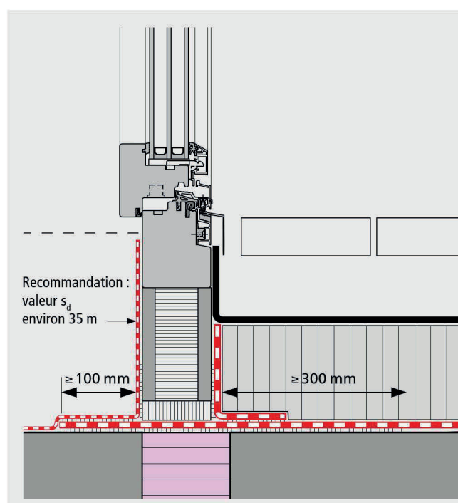
Figure 5.138: Raccordement au pare-vapeur des éléments de porte et de fenêtre avec console isolante.
