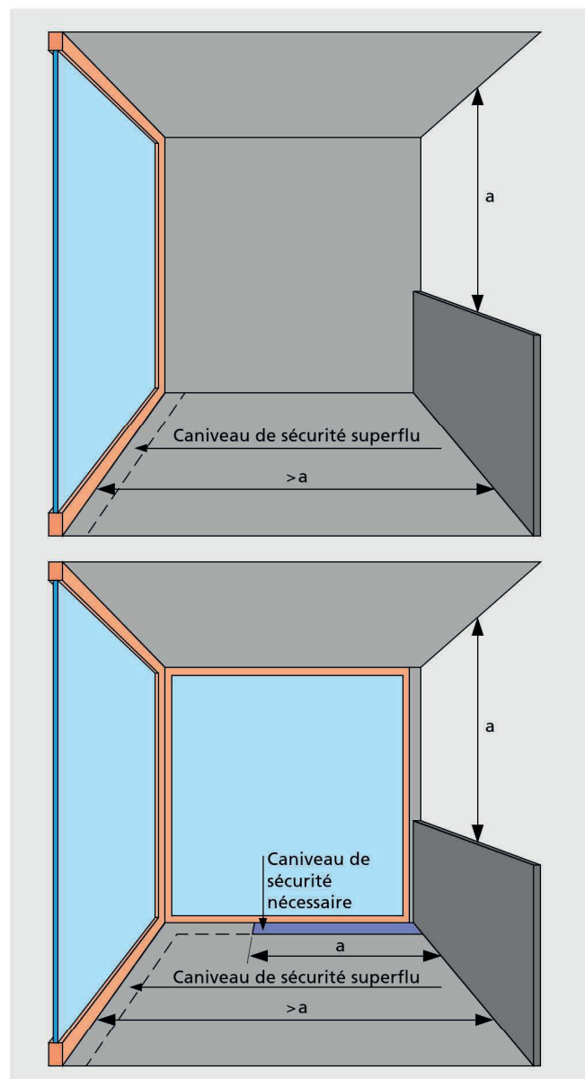
Figure 5.142: La nécessité d'un caniveau de sécurité dépend de la position du seuil par rapport à l'ouverture de la loggia, du balcon ou de la terrasse.
