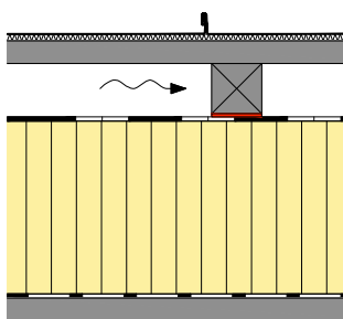
[FIG. 5] Comparaison des deux systèmes : pose homogène et non homogène.
