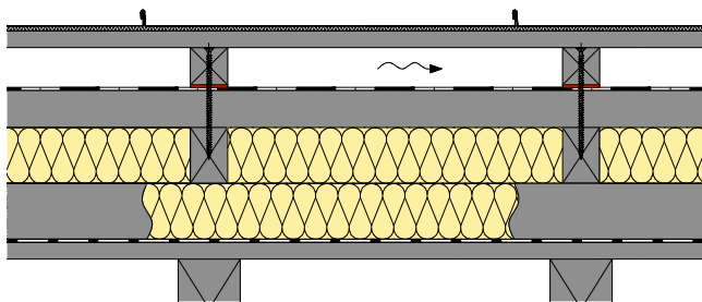
[FIG. 6] Combinaison : pose non homogène en haut, homogène en bas.
