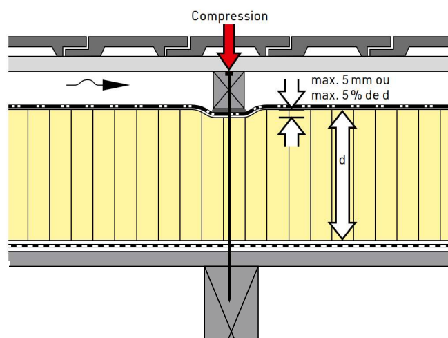
[FIG. 7] La déformation ne peut dépasser 5 % de l'épaisseur ou max. 5 mm.
