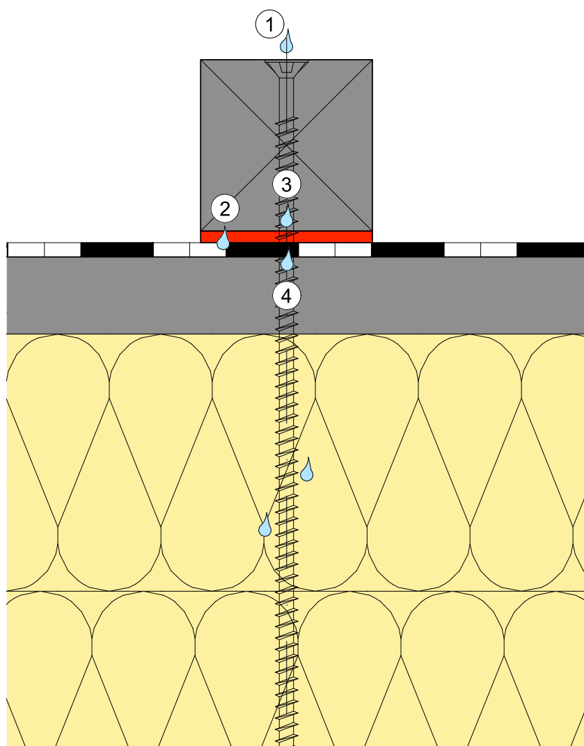
[FIG. 1] Infiltrations d'eau possibles au niveau des percements des moyens de fixation à travers les sous-couvertures.
