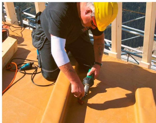
[FIG. 3] Soudage complet de la contre-latte.
